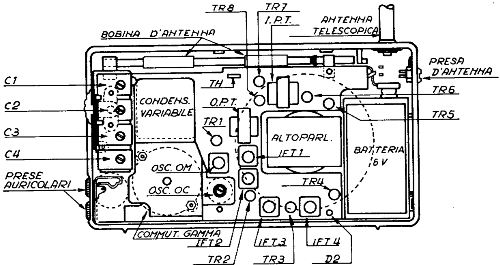
- Disposizione dei componenti sul pannello, entro la custodia.
